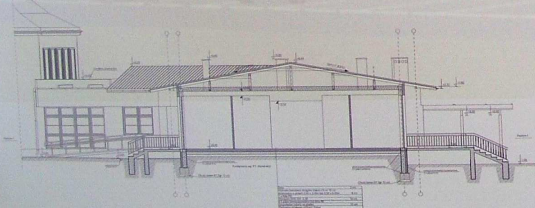
przekrój D-D
